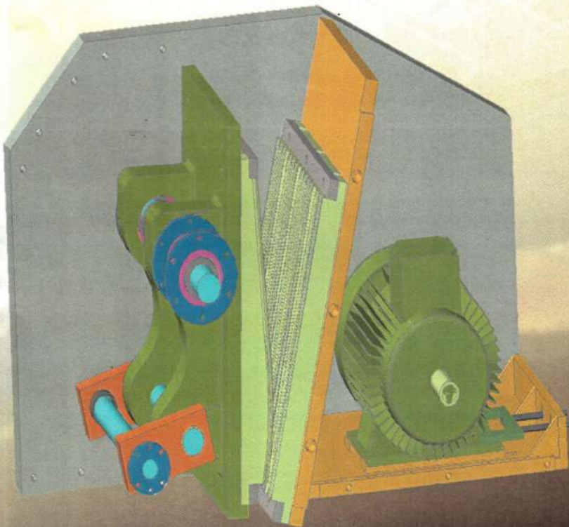
Moínho Maxilas Jaw Crusher
