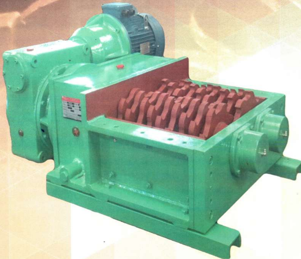
Moínho Destroçador de facas 317 Knives Crusher 317
